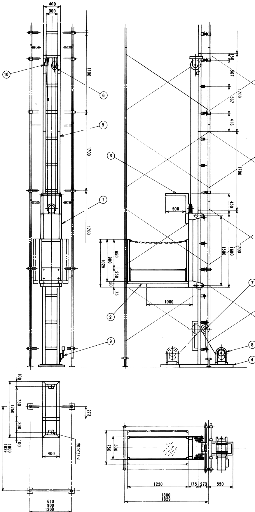
主要寸法図 単位：m/m
