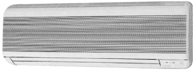
壁掛式エアコン (1馬力) 室内ユニット 寸法:W790×D174×H275mm 室外ユニット 寸法:W790×D250×H542mm
