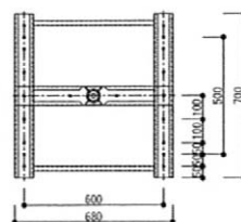
外形図
