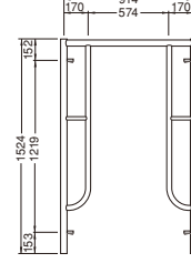
鳥居型簡易枠 A-305
