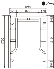
鳥居型建枠 A-4055B (1200SJ)
