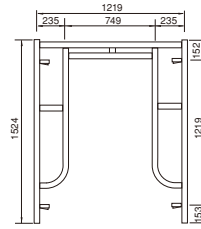
鳥居型建枠 A-405
