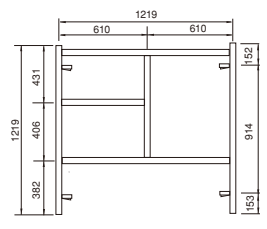
鳥居型建枠 A-404L
