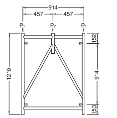
鳥居型建枠 AB-912
