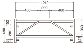
調節枠 A-417
