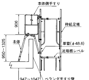
ベランダブリッジ
