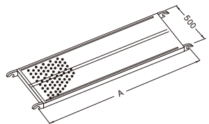
鋼製布板
