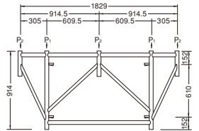
支保工ブラケット枠 AB-1809
