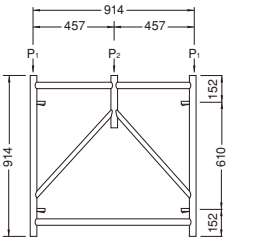
支保工ブラケット枠 AB-909
