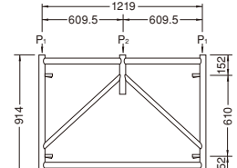
支保工ブラケット枠 AB-1209
