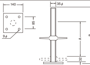
ジャッキベース(ミノ切)
