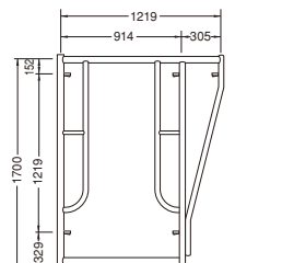
ブラケット枠 A-9117
