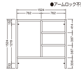
梯子型建枠 A-2(1500SJ)
