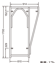
ブラケット枠 A-6117
