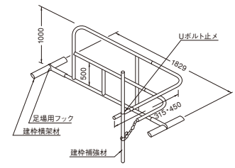
階段枠(アルミ製) AK-3055S
