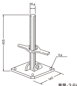
自在ジャッキベース
