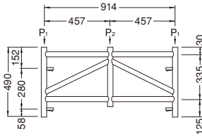
支保工ブラケット枠 AB-904
