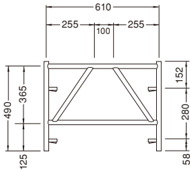
調節枠 AB-604
