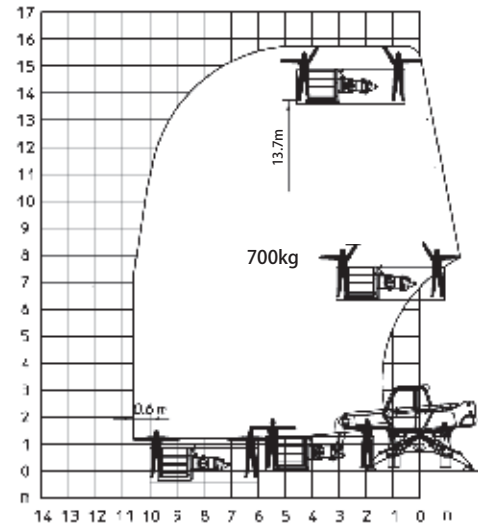
高所作業用ゴンドラ (PSE4400 700D)
