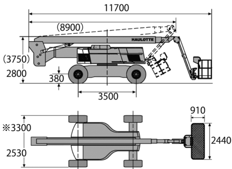
(mm) ( )輸送時寸法 ※アクスル張出時
