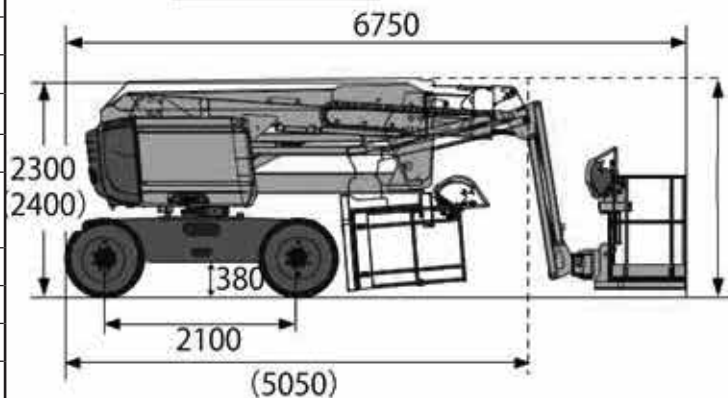
( )輸送時寸法
