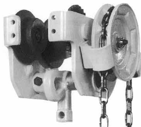
ギヤートロリー
