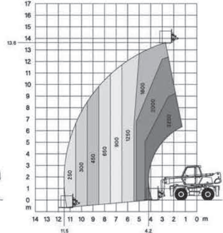
フォークアウトリガー未使用時
